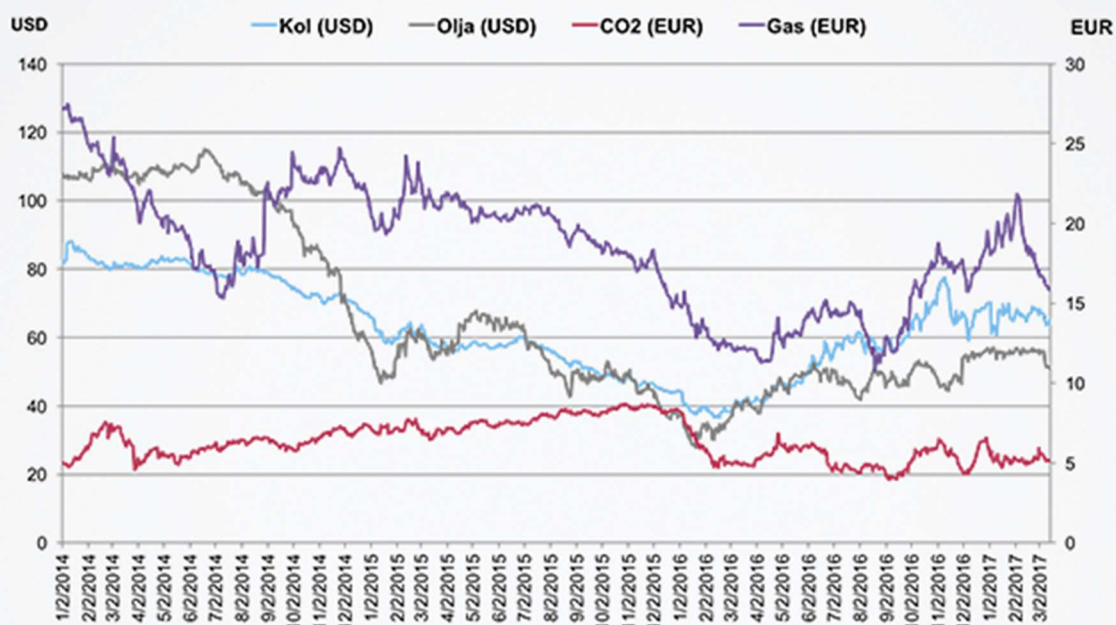
Råvarurpriser på gas, kol och utsläppsrätter för koldioxid
